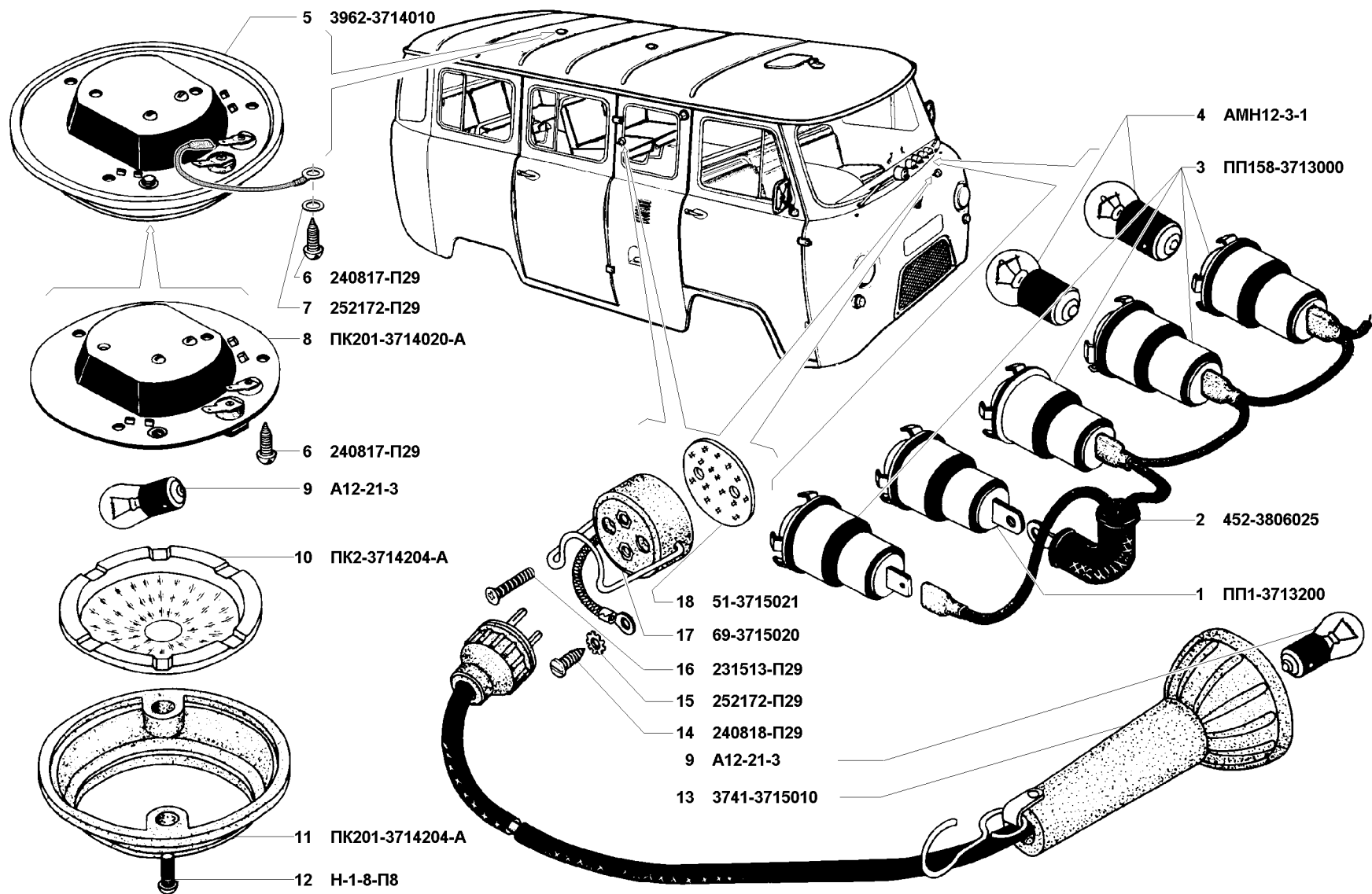
Рис. 104. Патроны ламп (3713), освещение кузова внутреннее (3714) и лампа переносная (3715)
